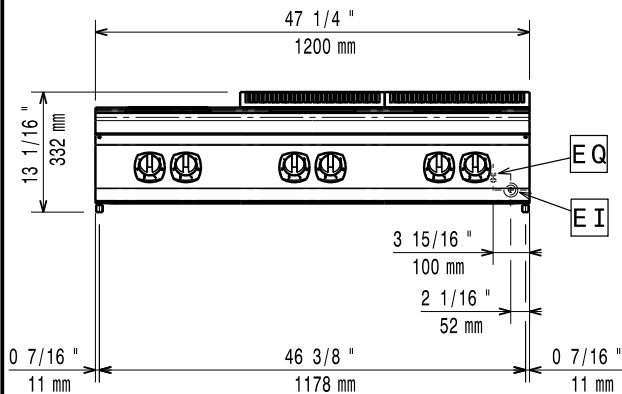
前视
